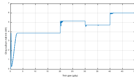
Hình 13. Công suất pin mặt trời
