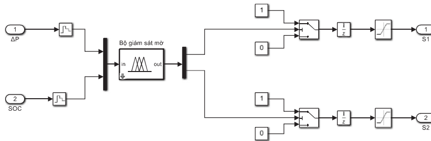
Hình 14. Bộ giám sát mờ trong Matlab Simulink
