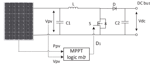
Hình 3. Bộ điều khiển MPPT logic mờ
