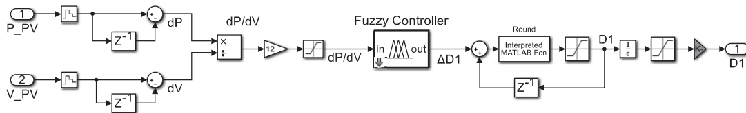
Hình 9. Bộ điều khiển MPPT logic mờ trong Matlab Simulink
