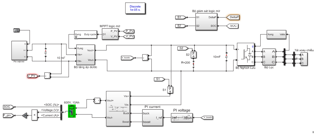
Hình 8. Mô phỏng trong Matlab Simulink
