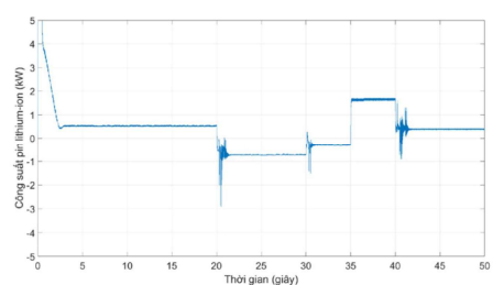
Hình 15. Công suất pin lithium-ion
