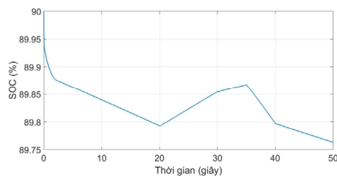
Hình 13. SOC của pin lithium-ion
