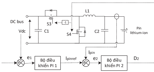
Hình 2. Bộ biến đổi hai chiều DC/DC
