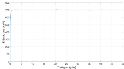
Hình 16. Điện áp Bus DC
