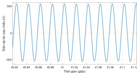
Hình 17. Điện áp tải xoay chiều
