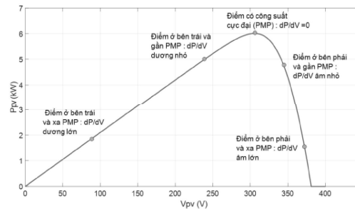
Hình 4. Điểm có công suất lớn nhất theo điện áp pin mặt trời
