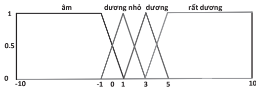
Hình 6. Hàm liên thuộc của biến đầu vào \Delta P (kW)
